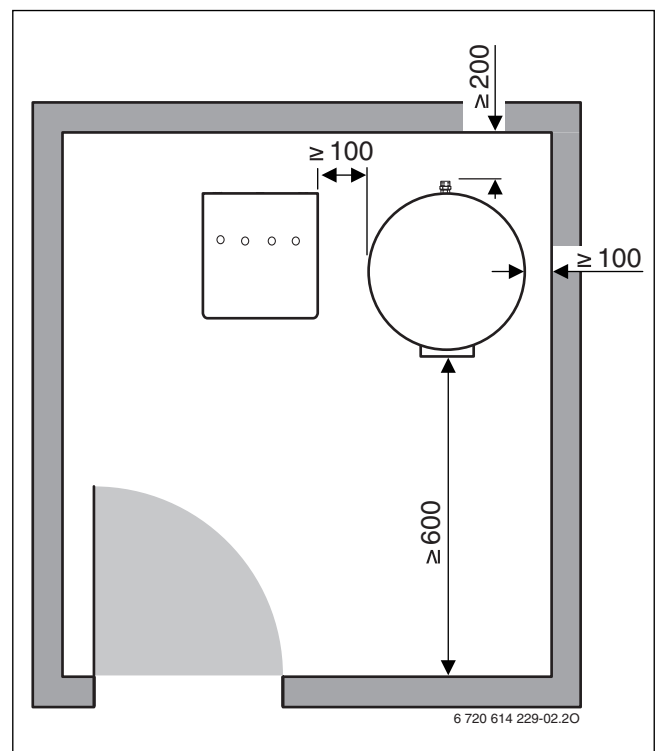
Fig. 2 Distâncias mínimas recomendadas em relação à parede
